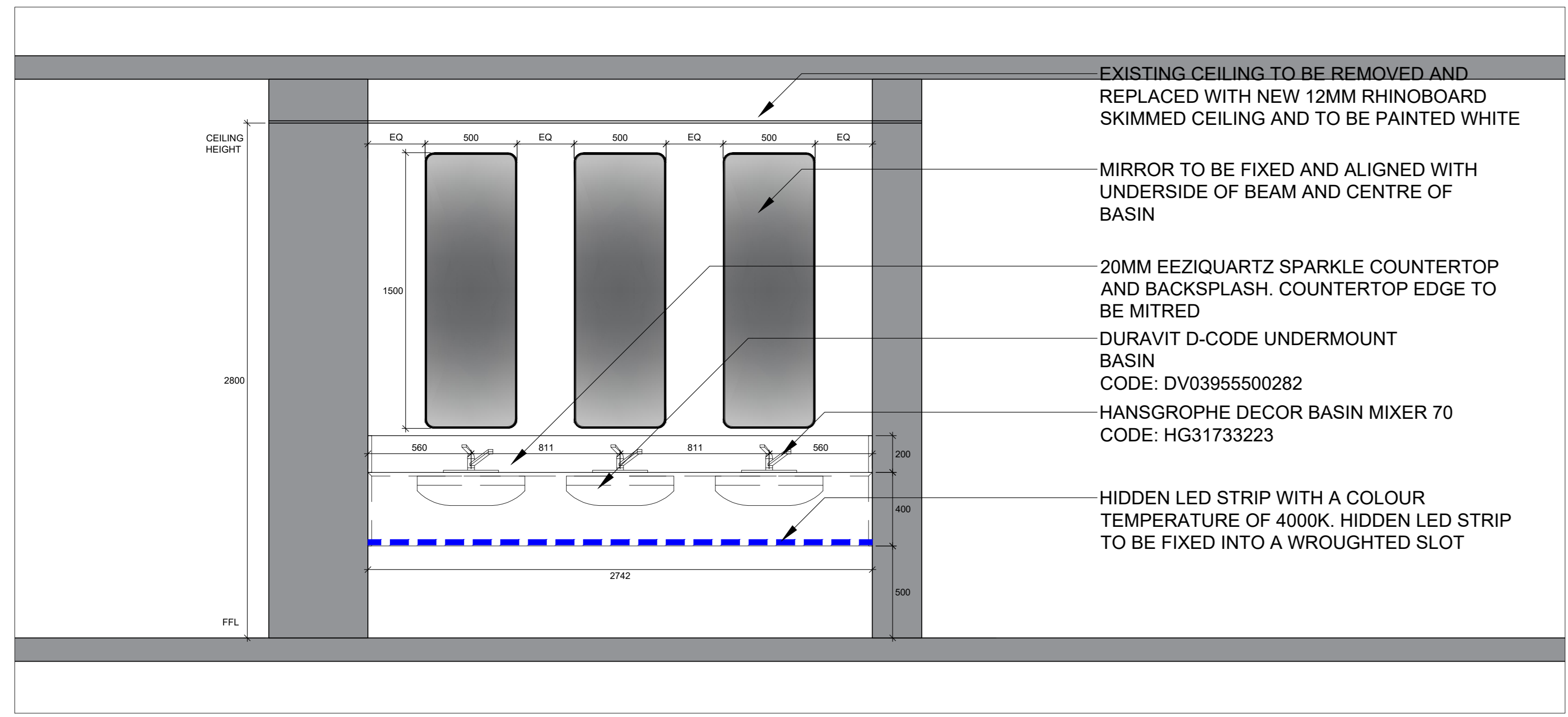
D. ELEVATION C-C SCALE 1:20
