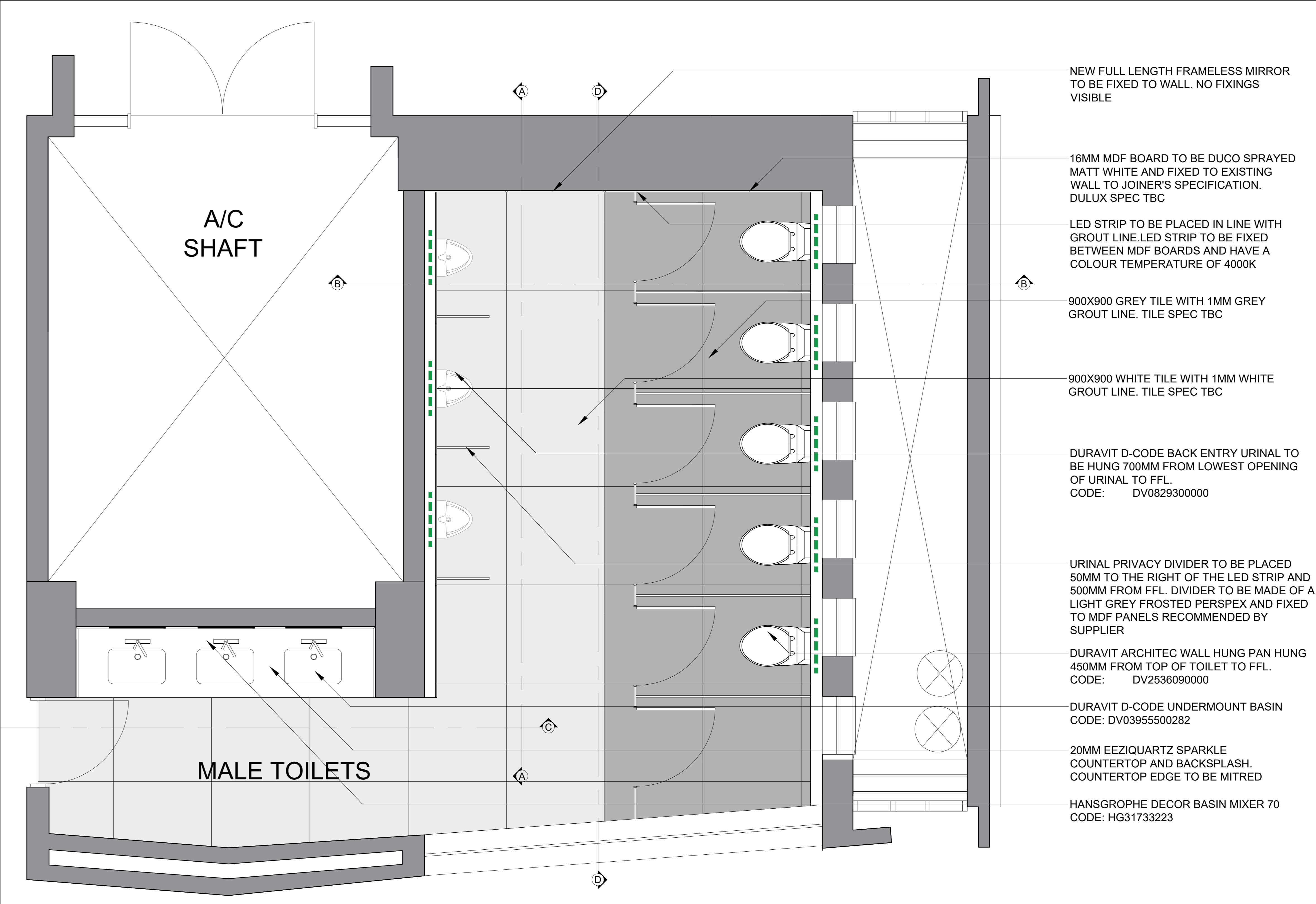
A. PLAN SCALE 1:30
