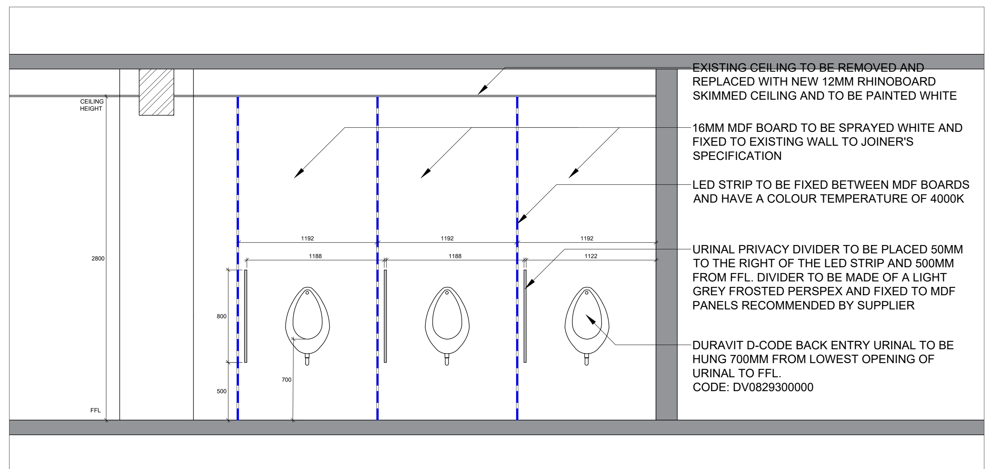
B. ELEVATION A-A SCALE 1:20
